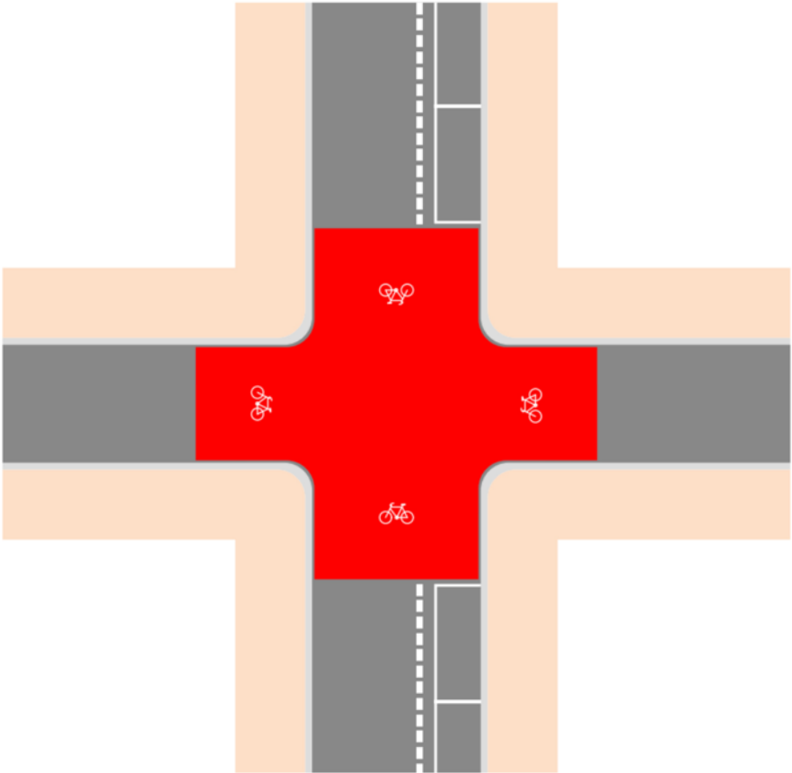
Abbildung 3: Knotenpunkte mit Vorfahrtssituation
